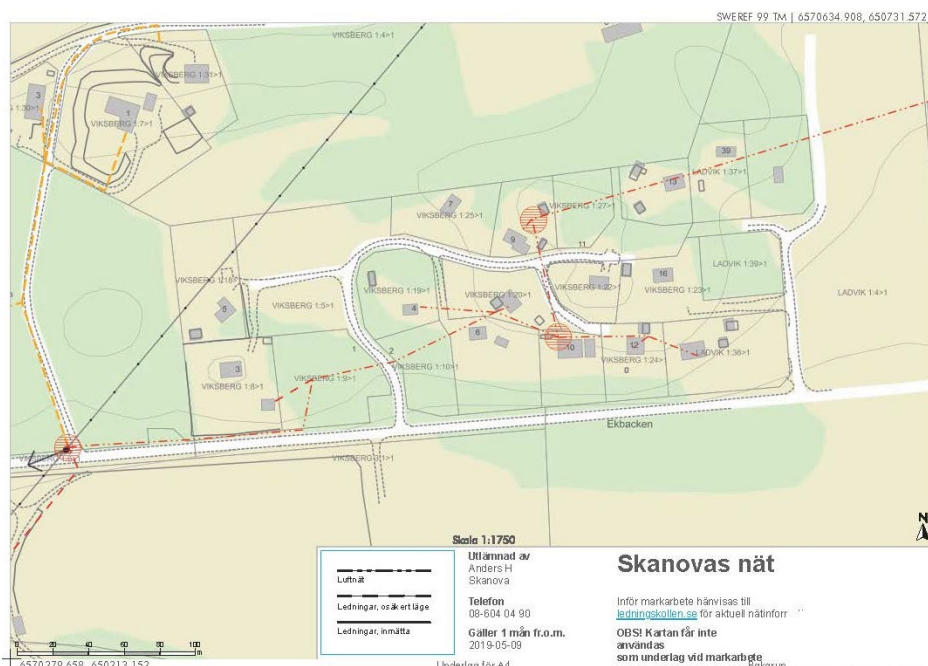
Figur 16. Skanovas nät.
