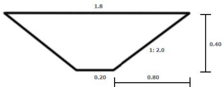
Figur 8. Principskiss över dimensionering av eventuella nya diken. Alla värden är angivna i meter (m) (StormTac, 2018). Dimensioneringen är gjord för att kunna hantera ett 10-årsregn med klimatfaktor.
