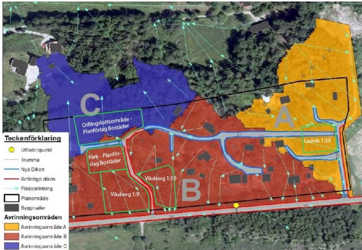
Figur 9. Bild med planområdets avrinningsområden med flödesriktningar och diken. Markerat med gröna linjer är odlingslottsområdet som ändrar användning till bostäder (inom avrinning C), parkområdet som ändrar användning till bostäder (inom avrinning B) och de tre fastigheterna som utgår från beräkningarna då de ej ingår i planförslaget/planområdet.
