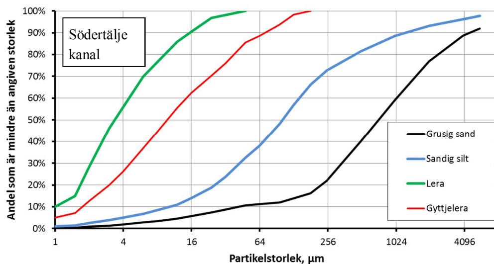
Figur 6. Typiska kornstorleksfördelningar för olika sedimenttyper från Mälaren (övre figur) och Södertälje kanal (nedre figur). Notera att skalan för x-axeln skiljer sig mellan figurerna.
