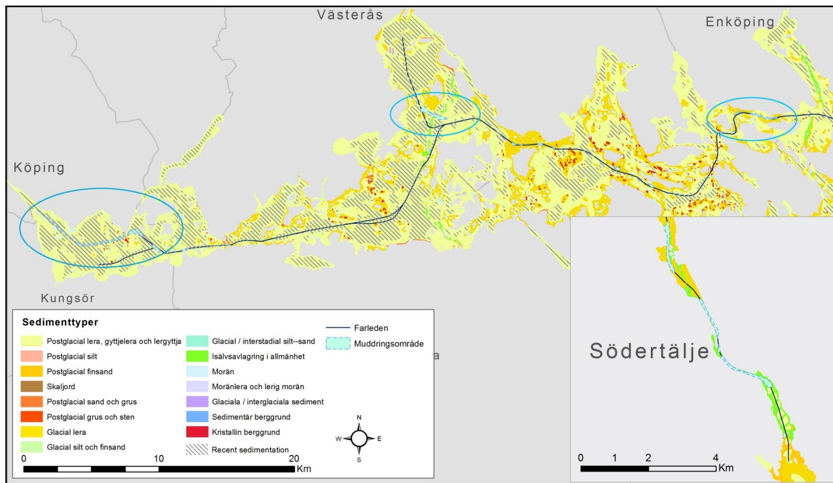
Figur 2. Sedimenttyper i västra Mälaren och Södertälje enligt SGU (©SGU). Ungefärlig utbredning av områden med pågående sedimentation av gyttjeler markeras med raster. De tre större muddringsområdena i Mälaren är noterade med ellipser.
