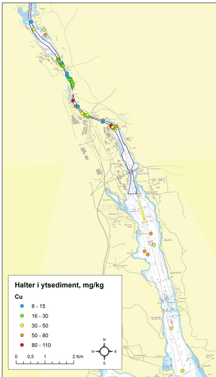
Figur 16. Kopparhalter i Södertälje kanals ytsediment. Halter anges per torrssubstans.
