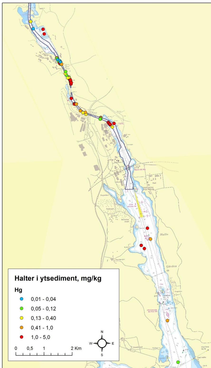
Figur 15. Kviksilverhalter i Södertälje kanals ytsediment. Halter anges per torrsubstans.
