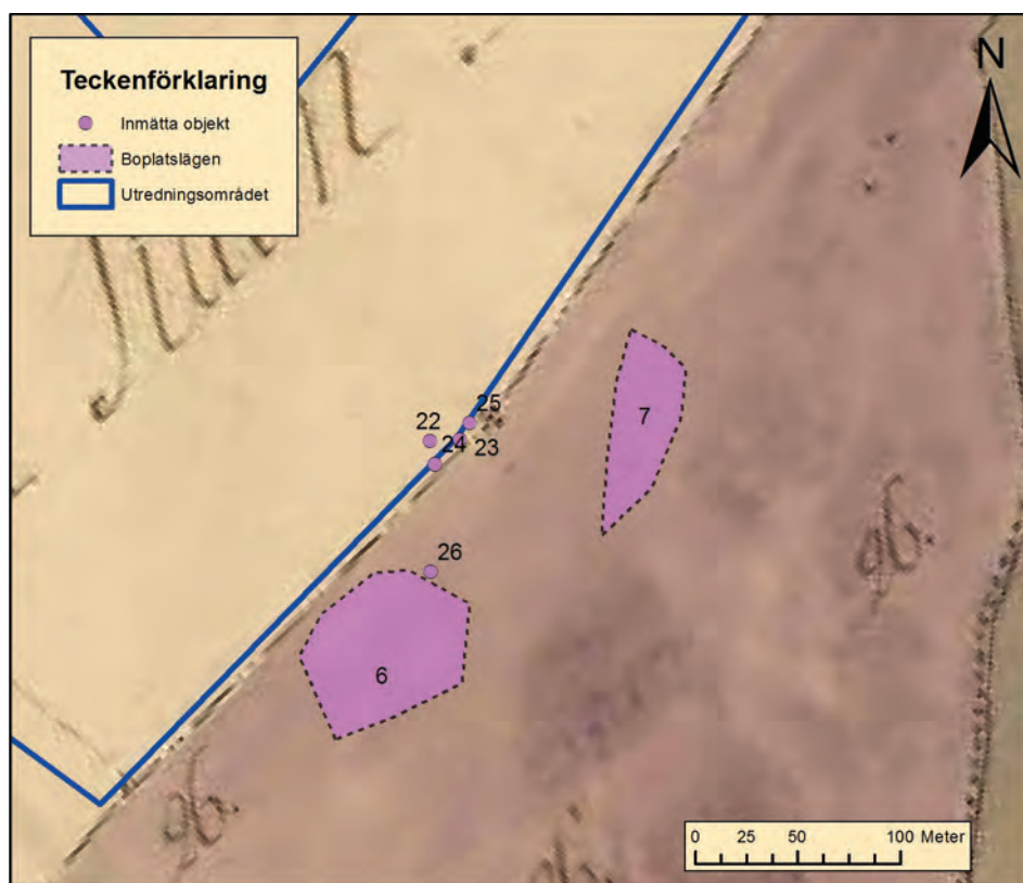
Figur 14. Gränsrösenas utritade på storskifteskartan från 1729. Rektifierad och i skala 1:4 000.
