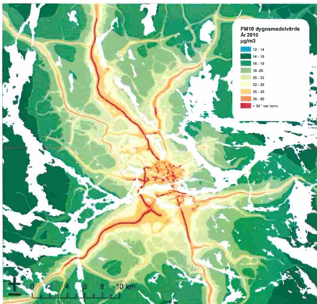
Figur 2.9. PM10 2010, dygnsmedelvärde mikrogram/m 3 . Rött illustrerar överskridande av miljökvalitetsnorm (MKN) över 50 mikrogram/m 3 . Gult indikerar att MKN kan överskridas. Målet ur hälsosynpunkt är 30 mikrogram/m 3 .
