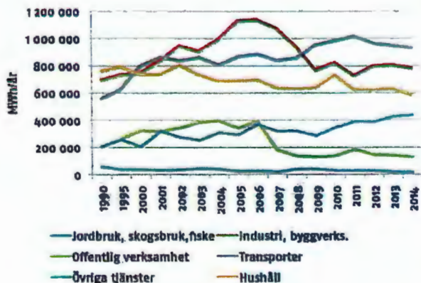
Slutlig energianvändning Södertälje 1990-2014 (MWh/år fördelat per sektor)
