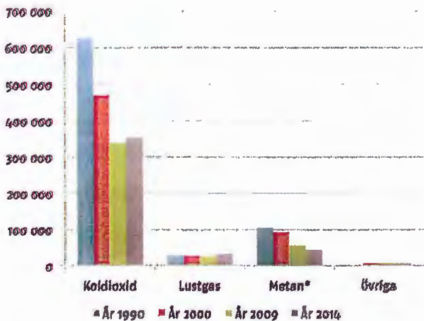
Utsläpp av växthusgaser i Södertälje 1990-2014 (ton CO2-ekvivalenter/år)
