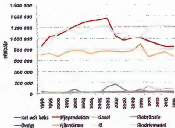
Slutlig energianvändning i Södertälje 1990-2014 fördelat per bränsle (MWh/år)
