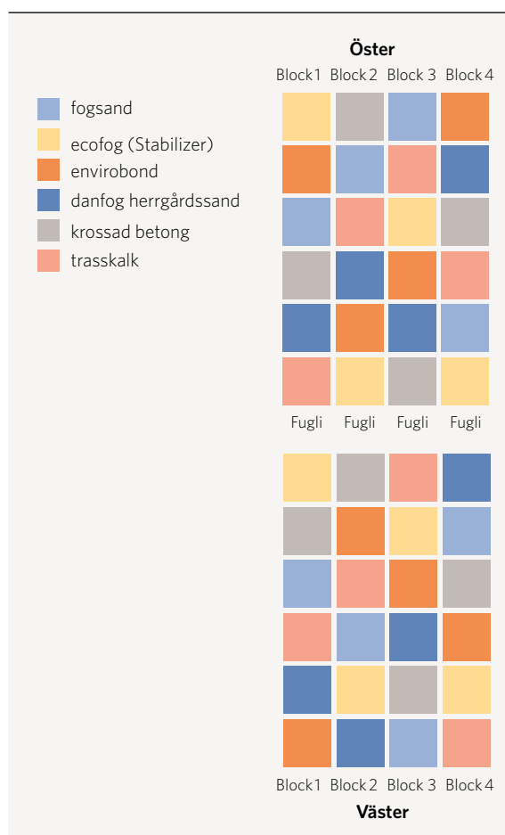
FIGUR 1. Försöksplan till försöket med olika fogmaterial
